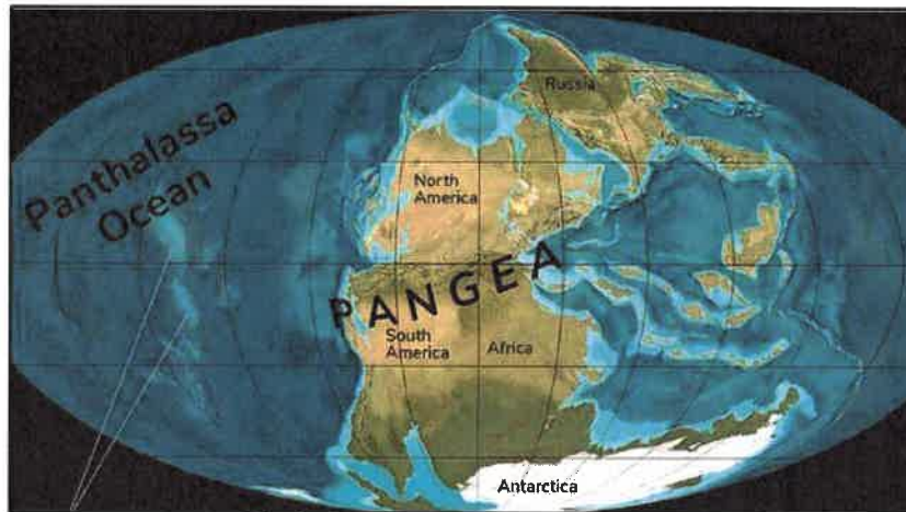
Fig. 3. Continentul și oceanul primordial (Sursa: https://www.geologypage.com )
