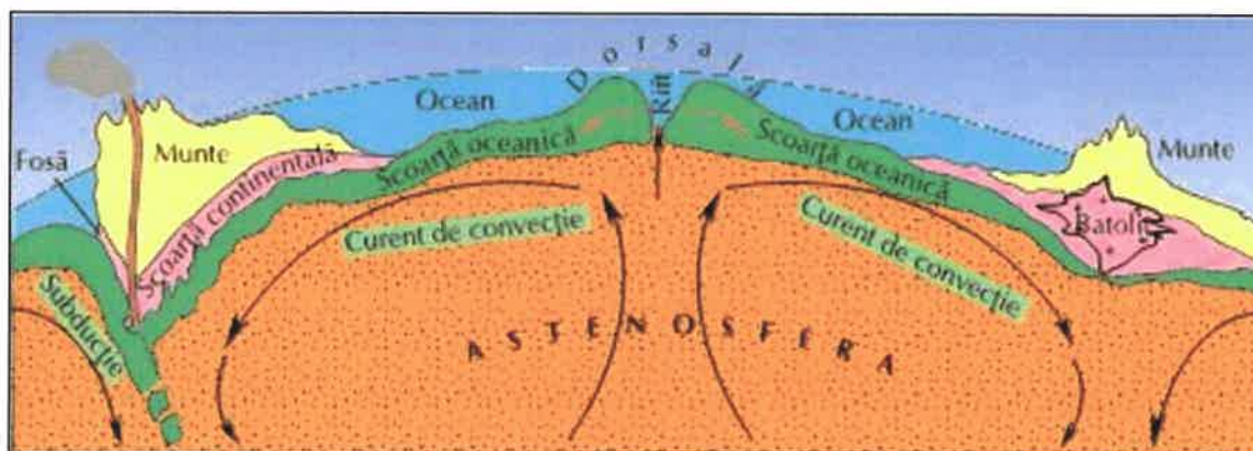
Fig. 1. Tectonica plăcilor – rift și subducție (Sursa: https://view.livresq.com/ )
